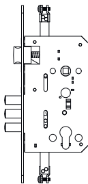
MPL 212 - P/N 26900251
